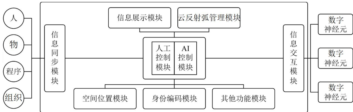
图 1 数字神经元功能模型
